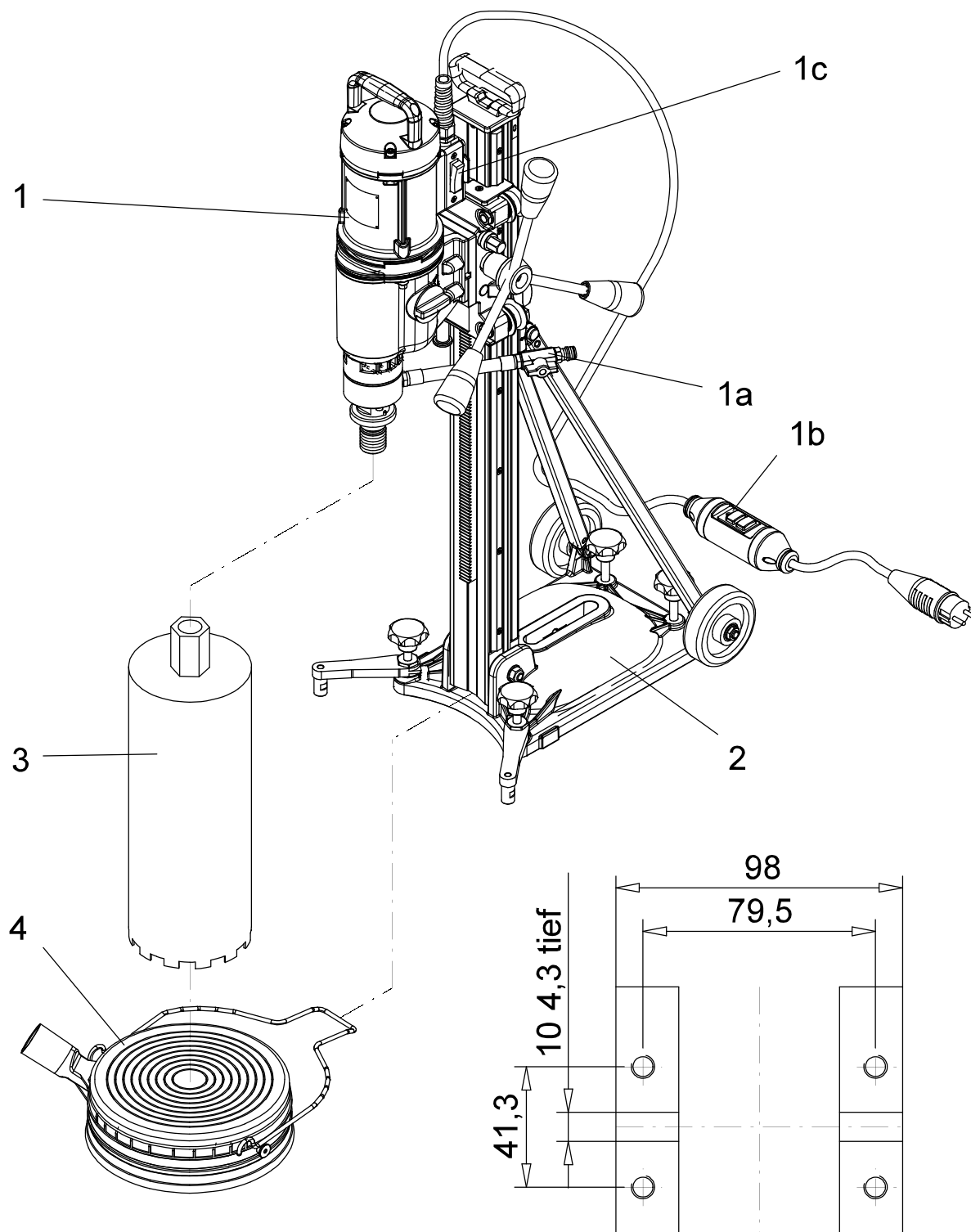
Maße - Getriebefuß
