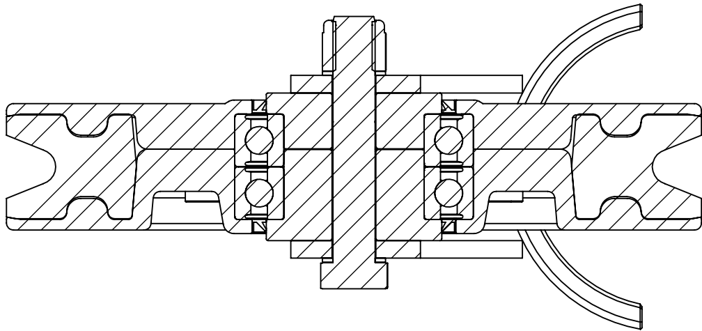
A-A
